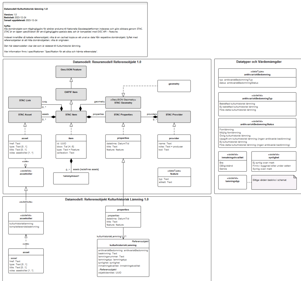
Figur 3: Datamodell för referensobjekt för informationsområde Kulturhistorik lämning, beskrivna i detalj i kapitel 5.2.1 till 5.2.5.
