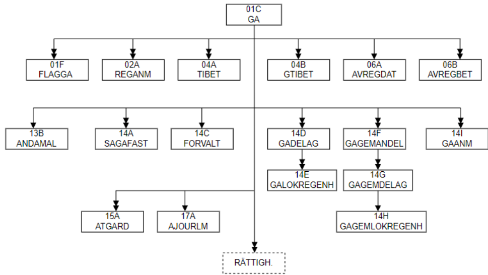
Figur 3. Beskriver relationerna mellan objekten i Gemensamhetsanläggning.
