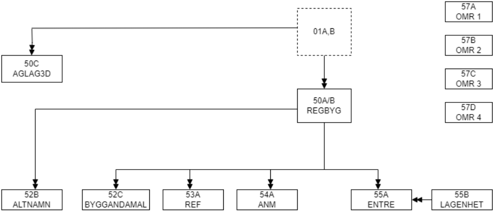
Figur 13. Beskriver relationerna mellan objekten i Byggnad.
