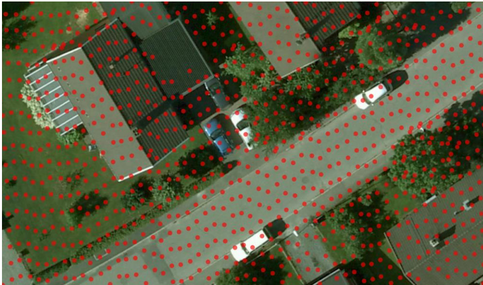
Figur 20. Ett exempel på hur glest laserträffarna (samtliga ekon) hamnar och den verkliga träffytan. På bilden syns också ett exempel på att punkter saknas över ett tak.
