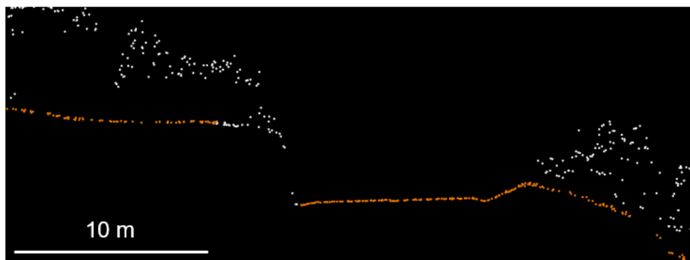
Figur 11. Bergvägg vid väg som inte har blivit klassad till mark, sannolikt p.g.a. den branta vinkeln. Profilen är dragen enligt det röda strecket i bilden nedan.
