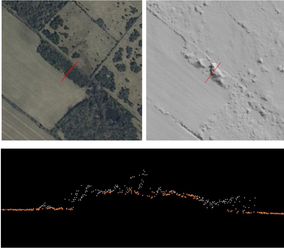
Figur 8. Täta låga buskage, som enbuskarna på Ölands alvar, kan vara redovisade som mark d v s små kullar i terrängmodellen. Eftersom inga laserpulser har trängt igenom buskaget till marken och buskarna har en "mjuk övergång" till marken uppfattas buskarna som mark vid den automatiska markklassningen.
