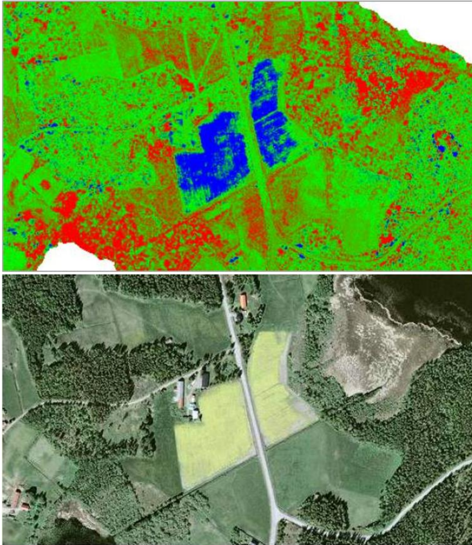
Figur 19. Överst detalj ur differensbild mellan två skanningar utförda vid olika årstider. Nederst ett ortofoto över samma terrängavschnitt. Uppe till höger ett område med vass, i mitten åkermark, och nere till vänster vass och annan låg vegetation. Differensbilden är grön vid 0 m skillnad och blir helt röd respektive blå vid \pm 0.4 m skillnad i höjd.
