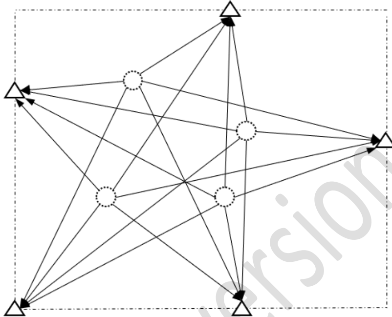
Figur 7. Exempel på terrestert 3D-nät som mäts in med totalstation från fria uppställningar. Konfigurationen utgörs av fyra ommarkerade uppställningar (ringar) och fem stompunkter (trianglar), vilket ger k = 0,52 i plan och k = 0,64 i höjd (se svarta rutor med vita siffror i Tabell 7 och Tabell 8).
