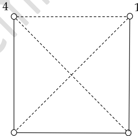
Figur 1. En session som mäts med fyra GNSS-mottagare har tre oberoende baslinjer (t.ex. 1-2, 2-3 och 3-4) och tre triviala (streckade). De triviala baslinjerna bör inte ingå i skattningen av nätets kontrollerbarhet.
