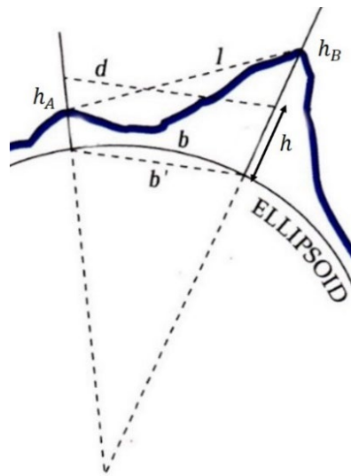
Figur 21. Lutnings- och höjdkorrektion vid längdmätning.
