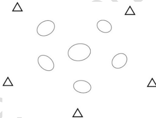
Figur 24. Redovisning av osäkerhetsellipser i ett plant stomnät. Utgångspunkterna – som betraktas som felfria – redovisas i form av trianglar.
