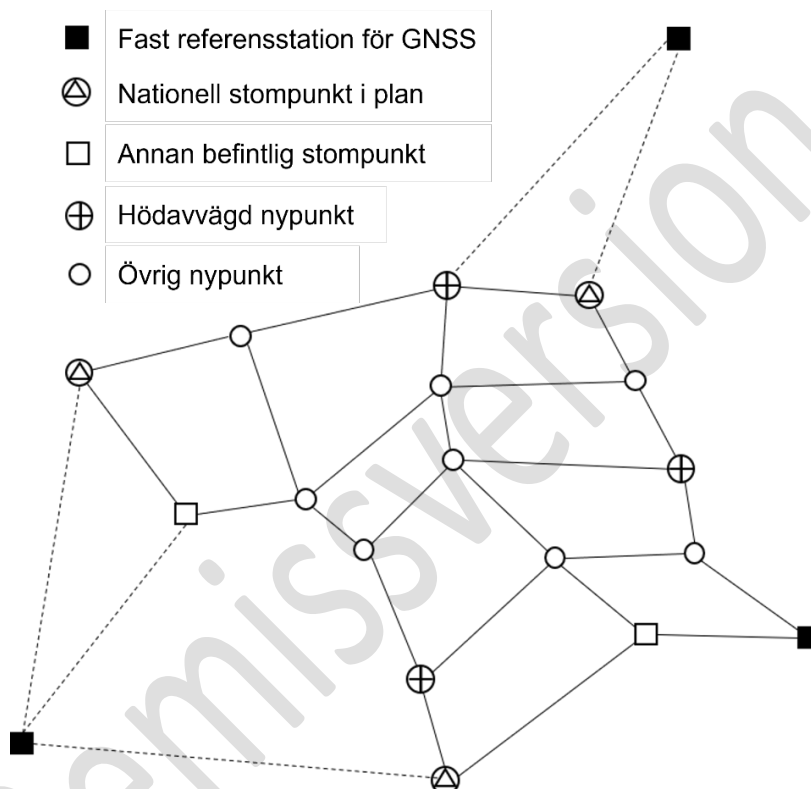
Figur 12. Exempel på hur ett GNSS-nät med huvudsakligen fyrsidiga former kan anslutas via olika utgångspunkter i plan respektive höjd.
