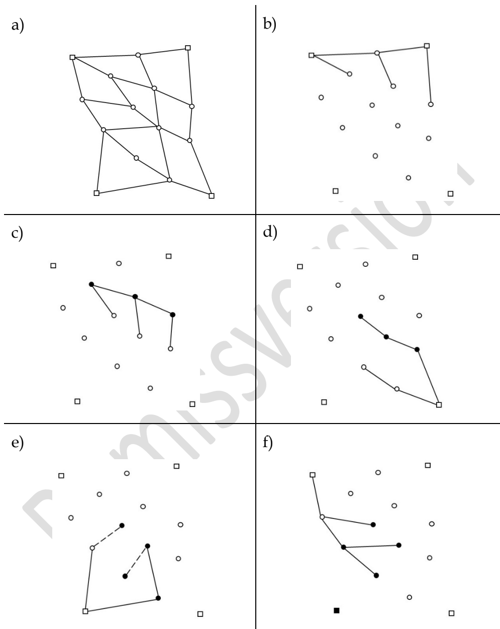
Figur 12. Ett GNSS-nät med oberoende baslinjer (a) ska mätas in med 6 st. GNSS-mottagare. Övriga figurer (b-f) visar hur mätningen kan utföras i fem sessioner, med fem oberoende baslinjer i varje session. Fyllda cirkular visar punkter där mottagare lämnas kvar. Observera att några "extra" oberoende baslinjer (streckade) erhålls i förhållande till nätsskissen i a).
