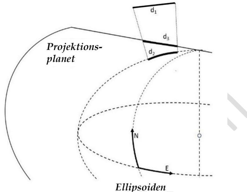
Figur 20. Mätt avstånd ( d_1 ) reduceras ner till avstånd på ellipsoiden ( d_2 ) genom höjdkorrektion. Därefter projiceras det vidare till avstånd i projektionsplanet ( d_3 ) med hjälp av en projektionskorrektion. Om d_1 = d_3 så tar de två korrektionerna ut varandra.
