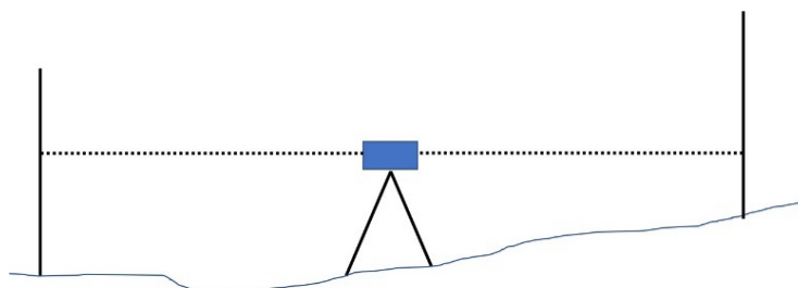
Figur 19. Genom att vid avvägning ställa upp instrumentet mitt emellan stängerna elimineras/reduceras inverkan från jordkrökning, refraction, kollimationsfel m.m.
