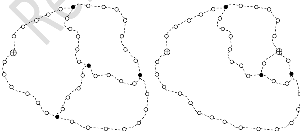
Figur 2. Vid etablering av höjdnät medför den tågformade geometrin att kontrollerbarhet och anslutning särskilt måste beaktas. Utgångspunkter visas som cirklar med kors och knutpunkter som fyllda cirklar.
