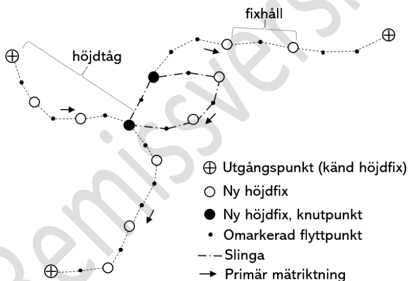
Figur 1. Principiell utformning av höjdnät: Mätningen mellan två höjdfixar utgör ett fixhåll och flera fixhåll bildar tillsammans ett höjdtåg. Höjdtågens ändar består av knutpunkter och/eller kända utgångspunkter i överordnat höjdnät.
