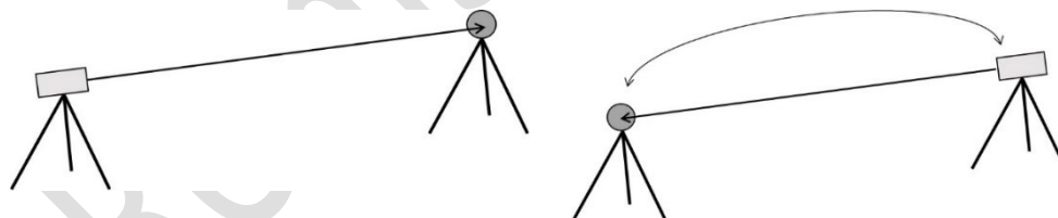
Figur 9. "Semi-korresponderande" trigonometrisk höjdmätning utförs från båda ändpunkterna – under likartade mätförhållanden och så nära varandra i tiden som möjligt. Tvångscentrering tillämpas och mätseriernas och mätperiodernas längd bör vara desamma som vid korresponderande mätning.
