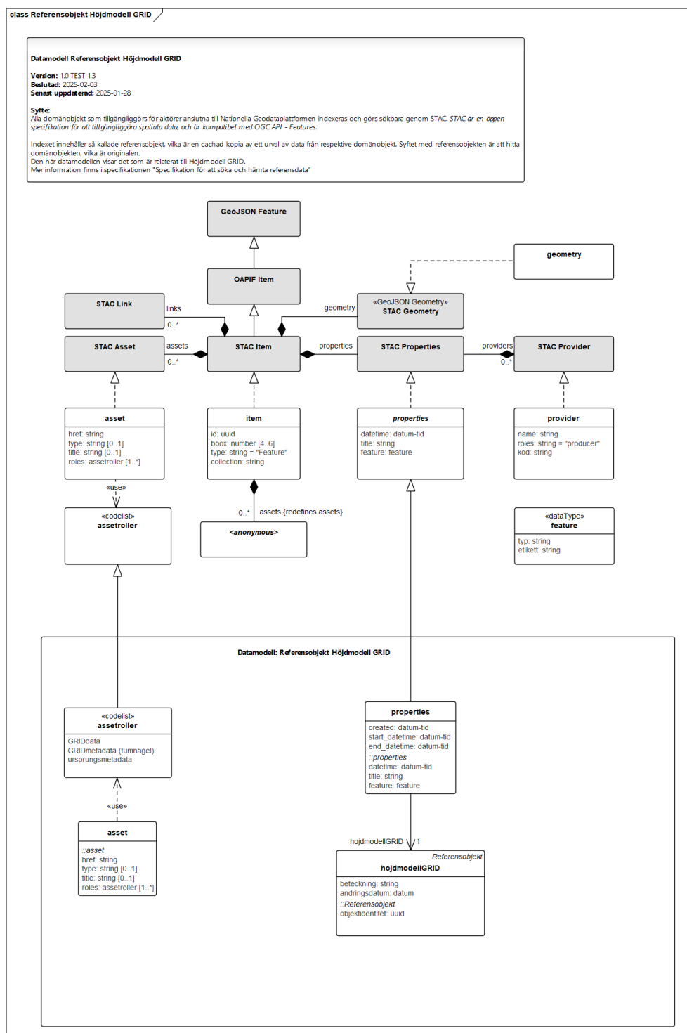
Figur 3: Datamodell för referensobjekt för informationsområde Höjdmodell GRID, beskrivet i detalj i kapitel 5.2.1 till 5.2.4.
